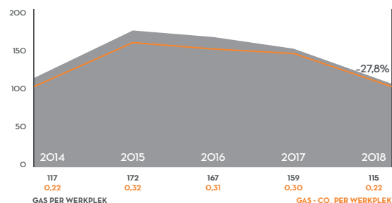
Energieverbruik gas per werkplek (in m 3 /CO 2 )
